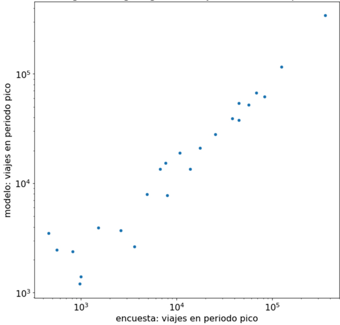
Illustration 16. Calibración de los flujos entre los municipios: regresión log / log
